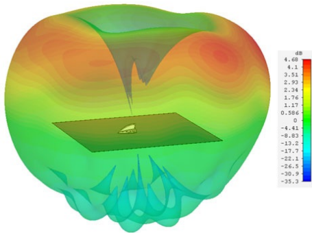
3D-GEWINNDARSTELLUNG SEITENANSICHT 4G-Element 700 MHz
