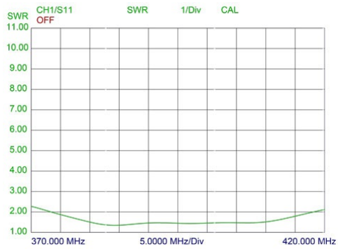
TYPISCHE SWR-KURVE INTEGRIERTES UHF *
